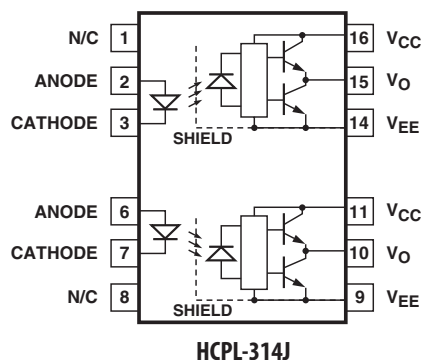
HCPL-314J
