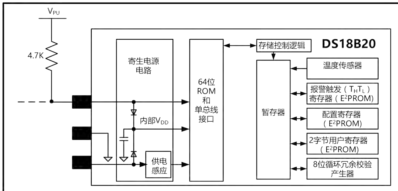
图 1 DS18B20 框图
