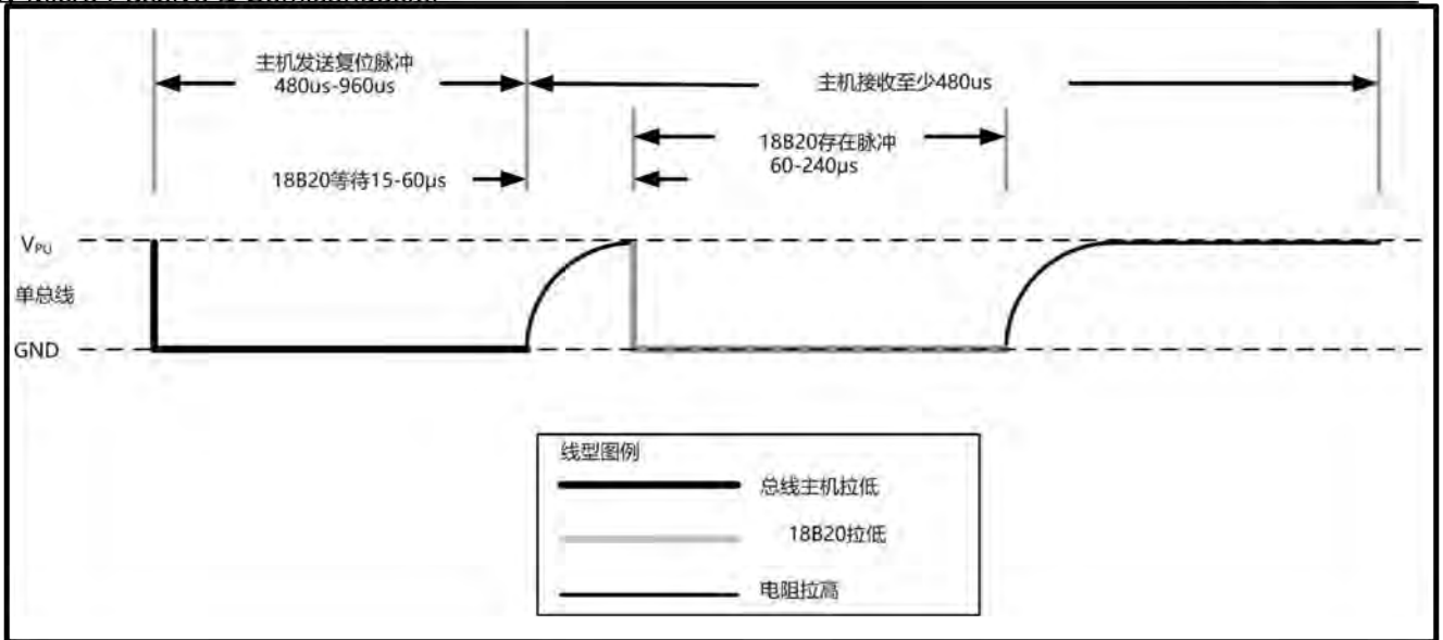
图 13 初始化时序
