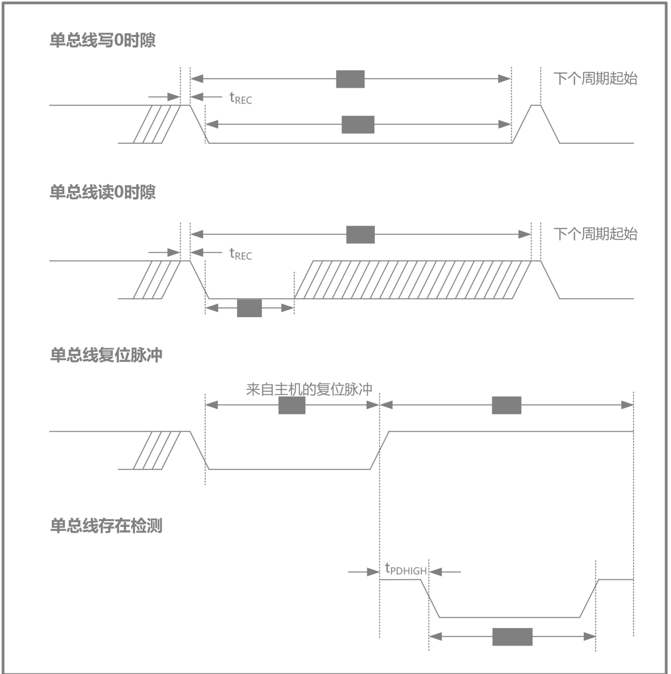
图 18 时序图
