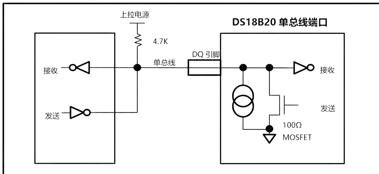
图 10 硬件配置
